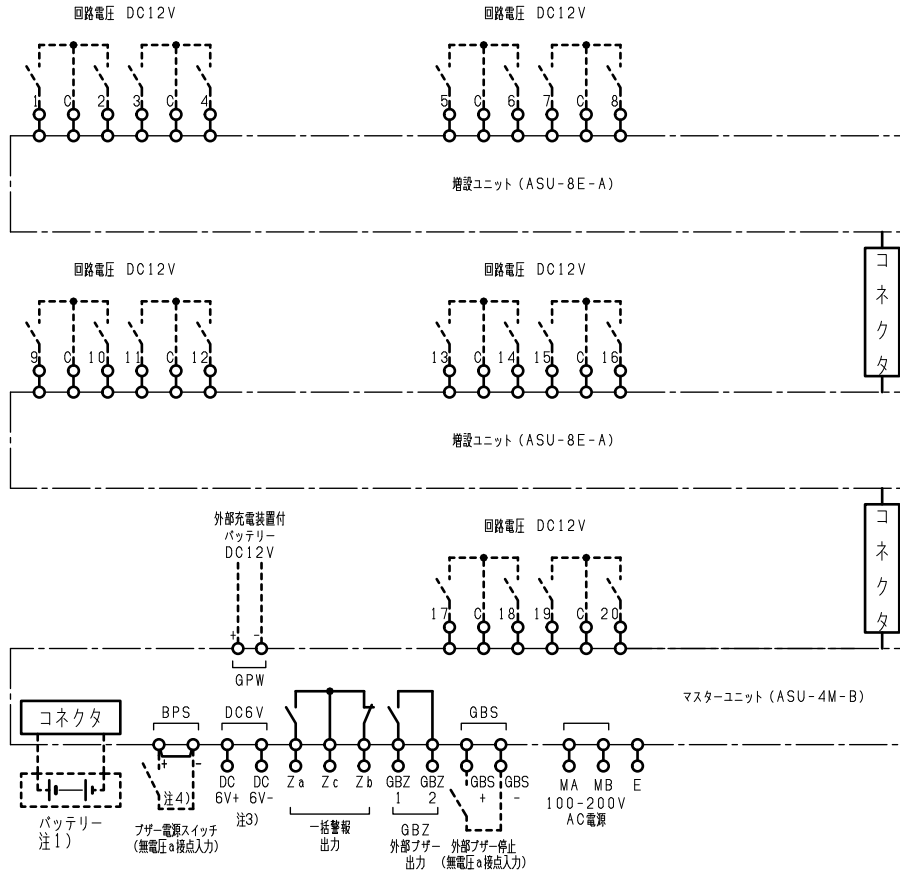
■回路図
