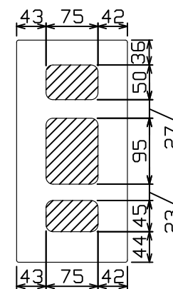
配線孔寸法図(//部開口)
