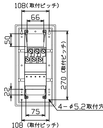
配線孔寸法図(//部開口)
