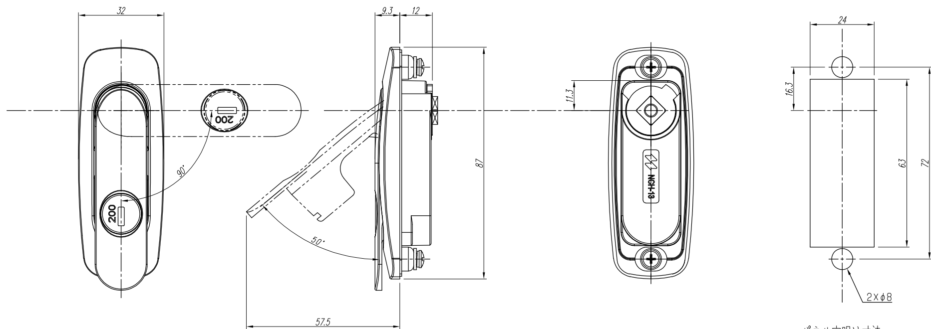
パネル穴明け寸法
