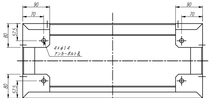
【DBP形電線固定金具使用可能範囲】
