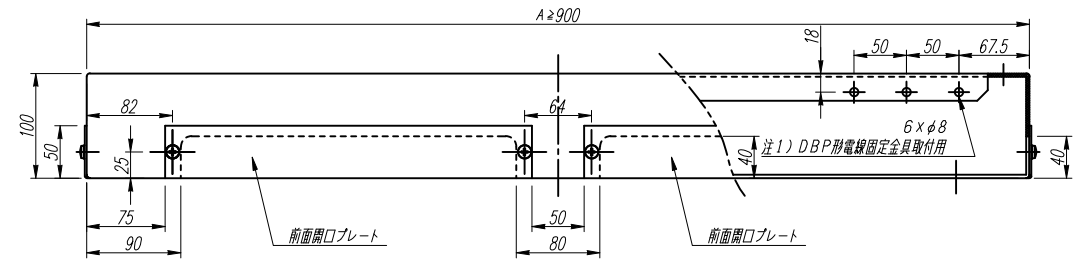
【DBP形電線固定金具使用可能範囲】
