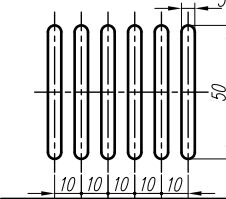
スリット部詳細図 (縮尺1/2)
